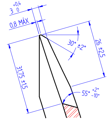
Detalhe C
